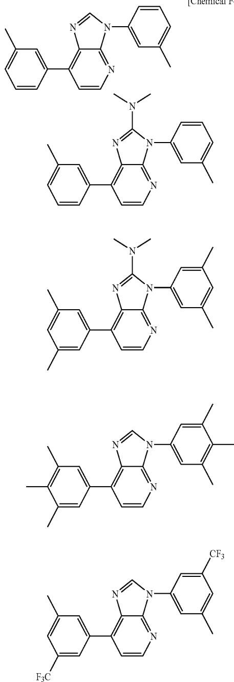
[Chemical Formulae 3]
